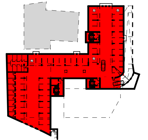
TIEFGARAGE - EBENE -01
